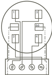
SSD-3W-6J SHD-3W-6J 4900-3W6J-G2 FORM 45
